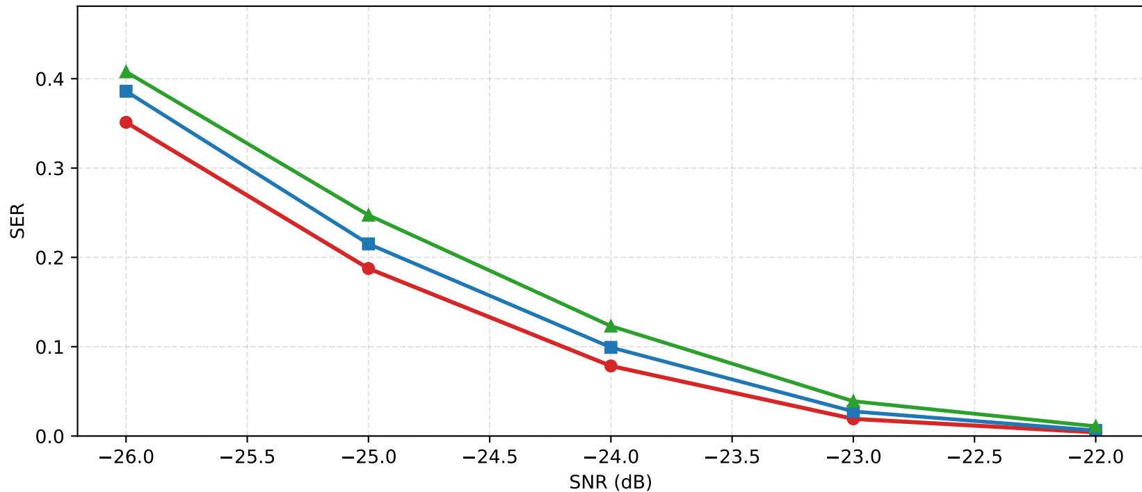
SER vs SNR: Phase-Line v2
